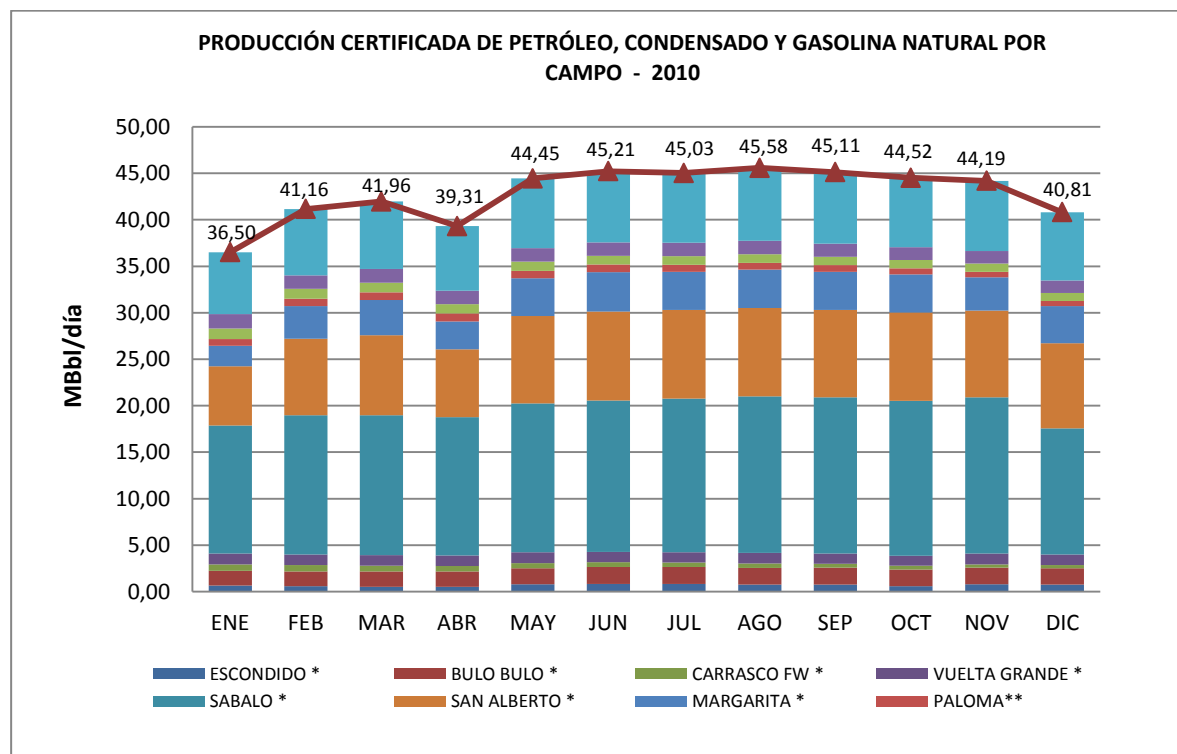
PRODUCCIÓN CERTIFICADA DE PETRÓLEO, CONDENSADO Y GASOLINA NATURAL POR CAMPO (MBbl/día) 2010
