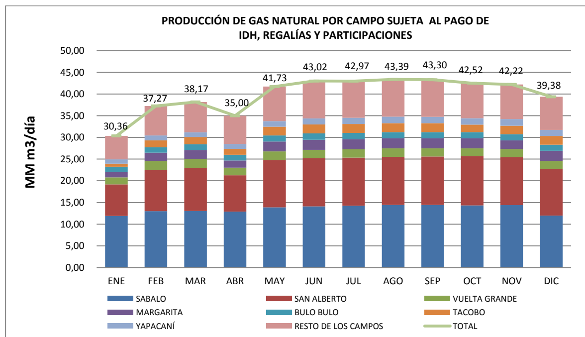
PRODUCCIÓN DE GAS NATURAL POR CAMPO SUJETA AL PAGO DE IDH, REGALÍAS Y PARTICIPACIONES (MMm3/día) 2010
