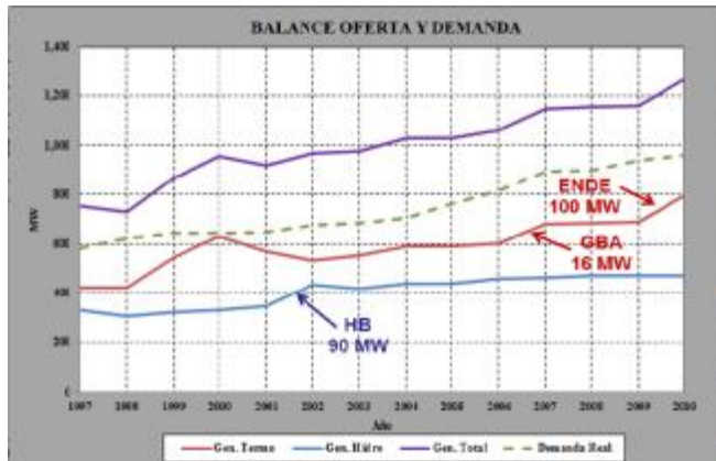
Gráfico 1.4. Capacidad de Generación vs Demanda Máxima del Sistema Boliviano.
