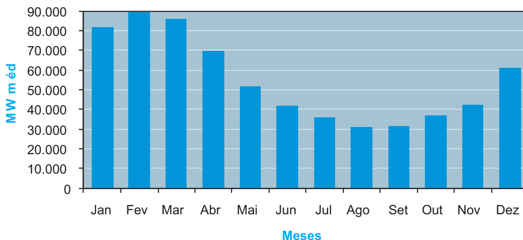
Gráfico 1 Energia Natural Afluente: média histórica anual (*)
