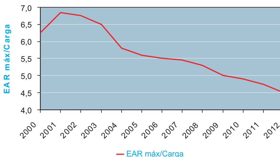
Gráfico 3 Evolução da capacidade de regularização dos reservatórios EAR - Energia Armazenada - Máxima Brasil sobre carga do SIN
