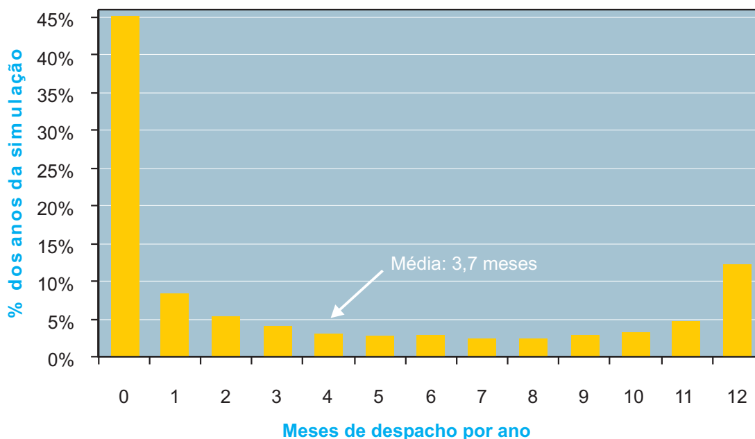
Gráfico 5 Meses de despacho por ano em simulação de dez mil anos Usina térmica com CVU de R$ 140/MWh
