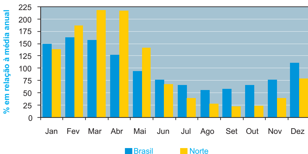
Gráfico 2 Energia Natural Afluente: comparação da média de longo termo entre Brasil e Região Norte. (em % da média anual)
