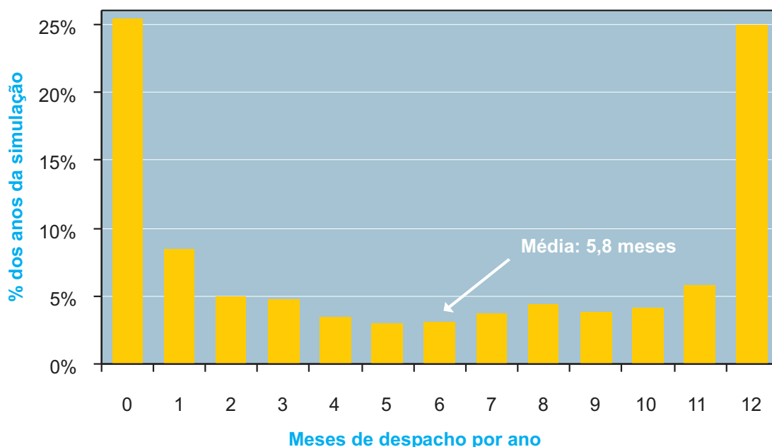
Gráfico 4 Meses de despacho por ano em simulação de dez mil anos Usina térmica com CVU de R$ 90/MWh
