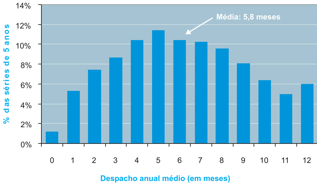
Gráfico 7 Despacho médio em meses por ano. Simulação de duas mil séries de cinco anos. Térmica com CVU de R$ 90/MWh
