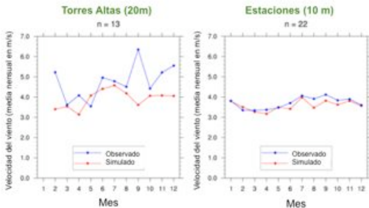
Figura 5: Ciclo estacional de la media mensual de velocidad del viento para datos simulados y observados correspondiente a: la velocidad del viento a 20 m en 13 torres altas (promedio - izquierda) y la velocidad del viento a 10 metros en 22 estaciones meteorológicas (promedio - derecha). La unidad de medida es metro por segundo (m/s).
