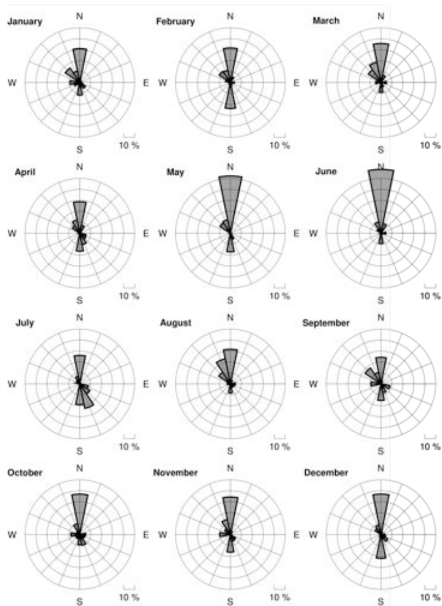
Figura III-37: Observado en SLJE (San José de Chiquitos, Bolivia)
