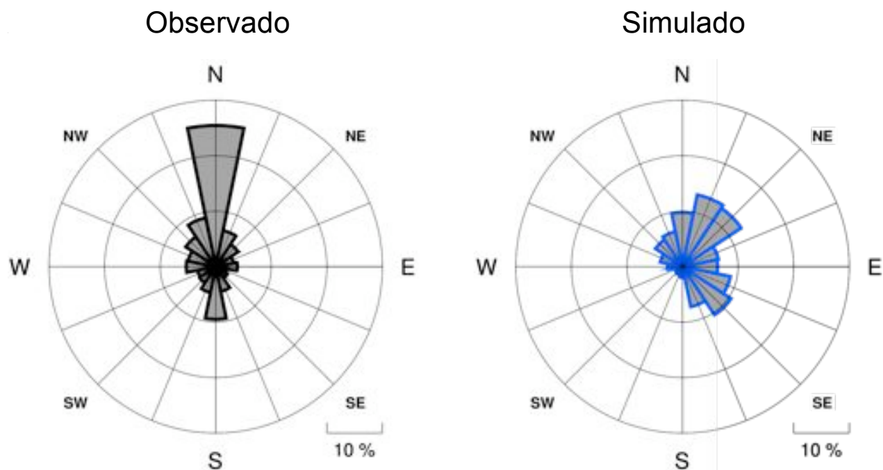
Figura III-2: Comparación Anual de Rosas de Viento: SBRB
