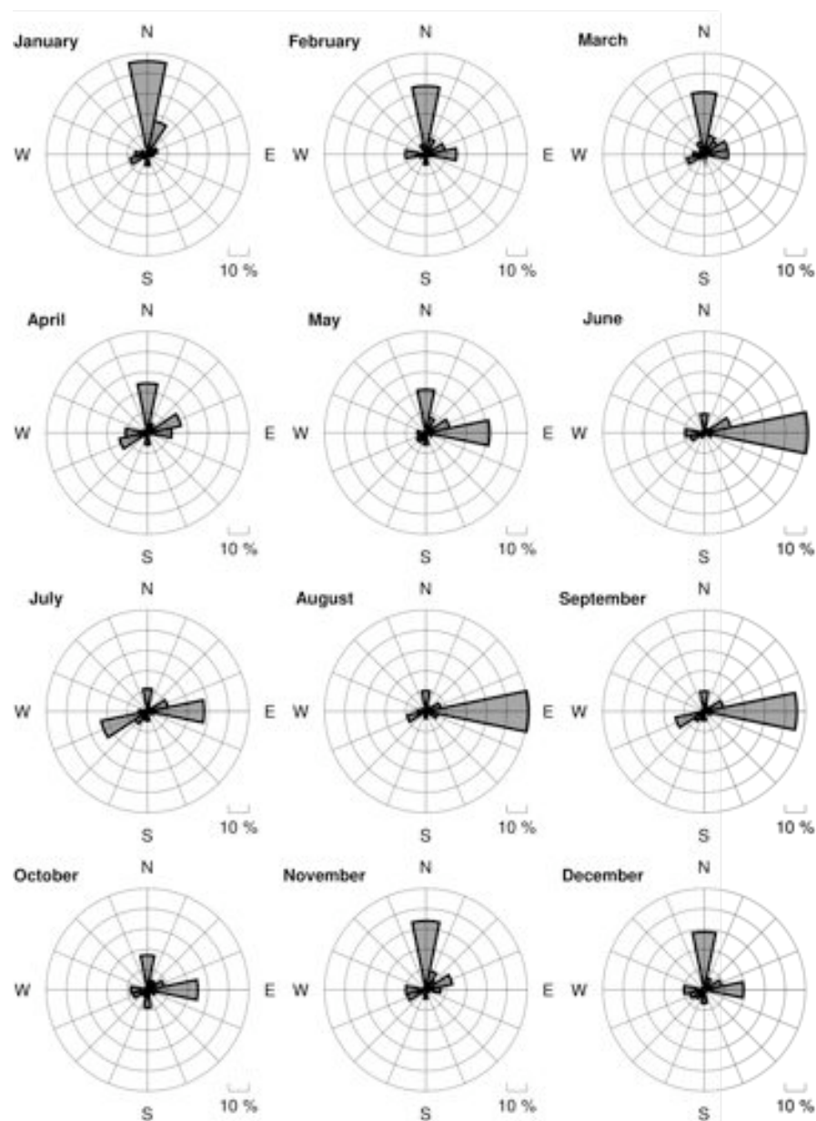
Figura III-47: Observado en SLPS (Puerto Suárez, Bolivia)
