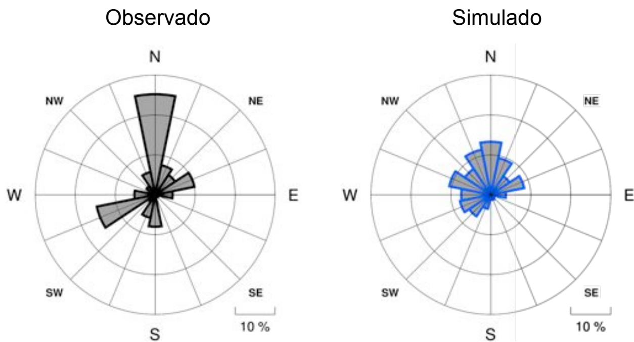
Figura III-12: Comparación Anual de Rosas de Viento: SLPO
