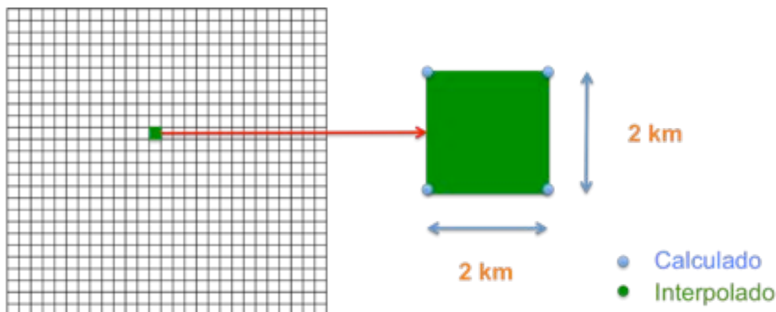
Figura 8: La gráfica arriba muestra la resolución horizontal de la simulación PNT utilizada para crear el Atlas Eólico de Bolivia. El modelo WRF calcula cifras meteorológicas discretas (velocidad del viento, temperatura, presión atmosférica, etc.) para cada esquina de cada celda en la grilla de 2 km x 2 km. Al iniciar la simulación 3TIER atribuyó a cada punto de la grilla información sobre uso de suelo, elevación y rugosidad.
