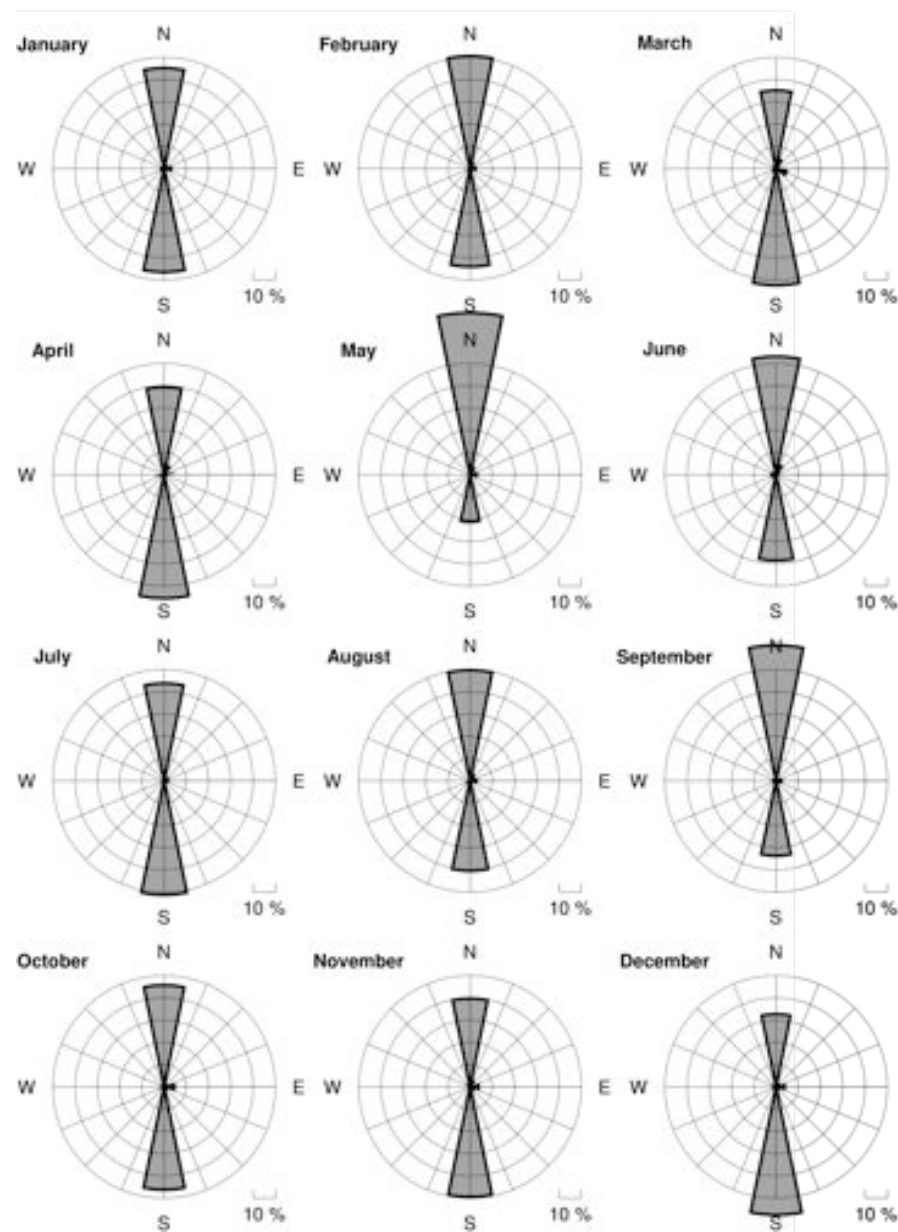
Figura III-65: Observado en SLYA (Yacuiba, Bolivia)
