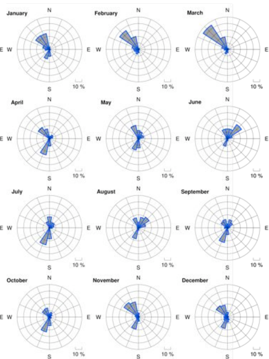
Figura III-48: Simulado en SLPS (Puerto Suárez, Bolivia)
