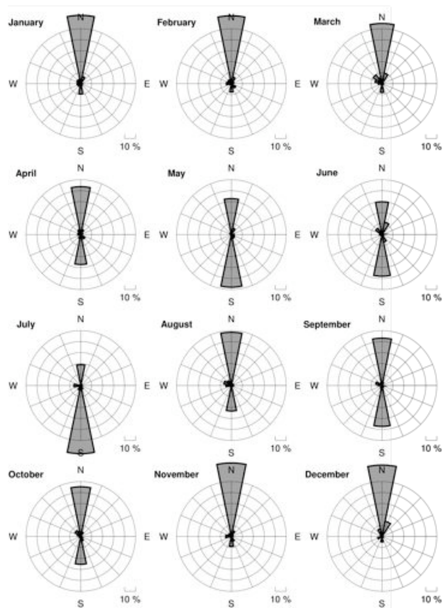
Figura III-51: Observado en SLRI (Riberalta, Bolivia)
