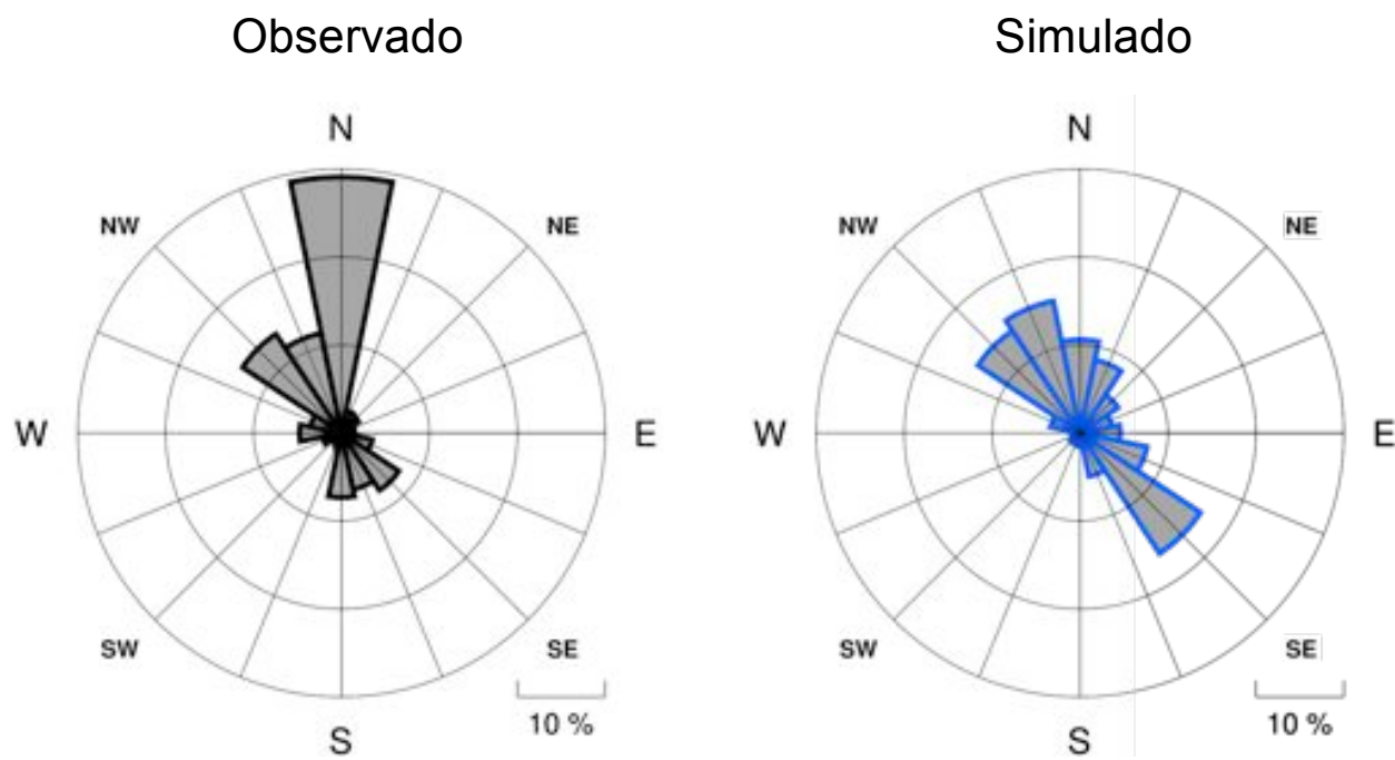
Figura III-5: Comparación Anual de Rosas de Viento: SLCO
