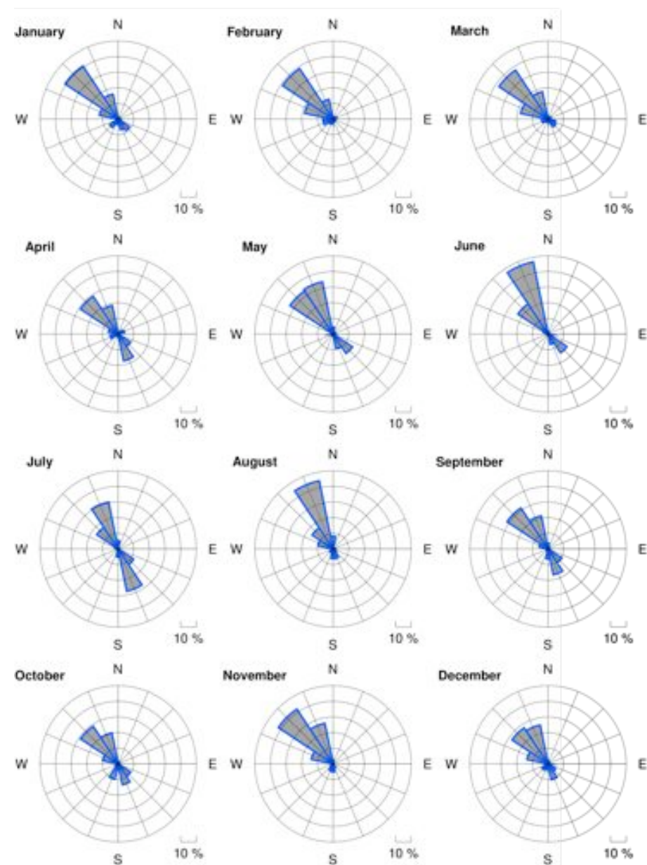
Figura III-34: Simulado en SLCP (Concepción, Bolivia)
