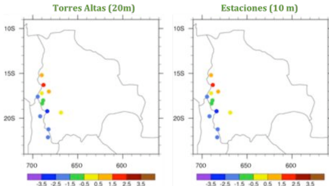
Figura 3: Mapas de diferencias entre velocidades del viento simuladas y observadas para las observaciones recolectadas en torres altas de 20 m (izquierda) y para las observaciones recolectadas en estaciones meteorológicas a 10 m (derecha). La unidad de medida es metro por segundo (m/s) y cada color representa el rango de sesgo mostrado en la leyenda al pie de la figura. Por ejemplo, puntos amarillos representan sitios de validación en los cuales los vientos simulados por 3TIER estuvieron entre 0.5 m/s menor y 0.5 m/s mayor a los vientos observados.
