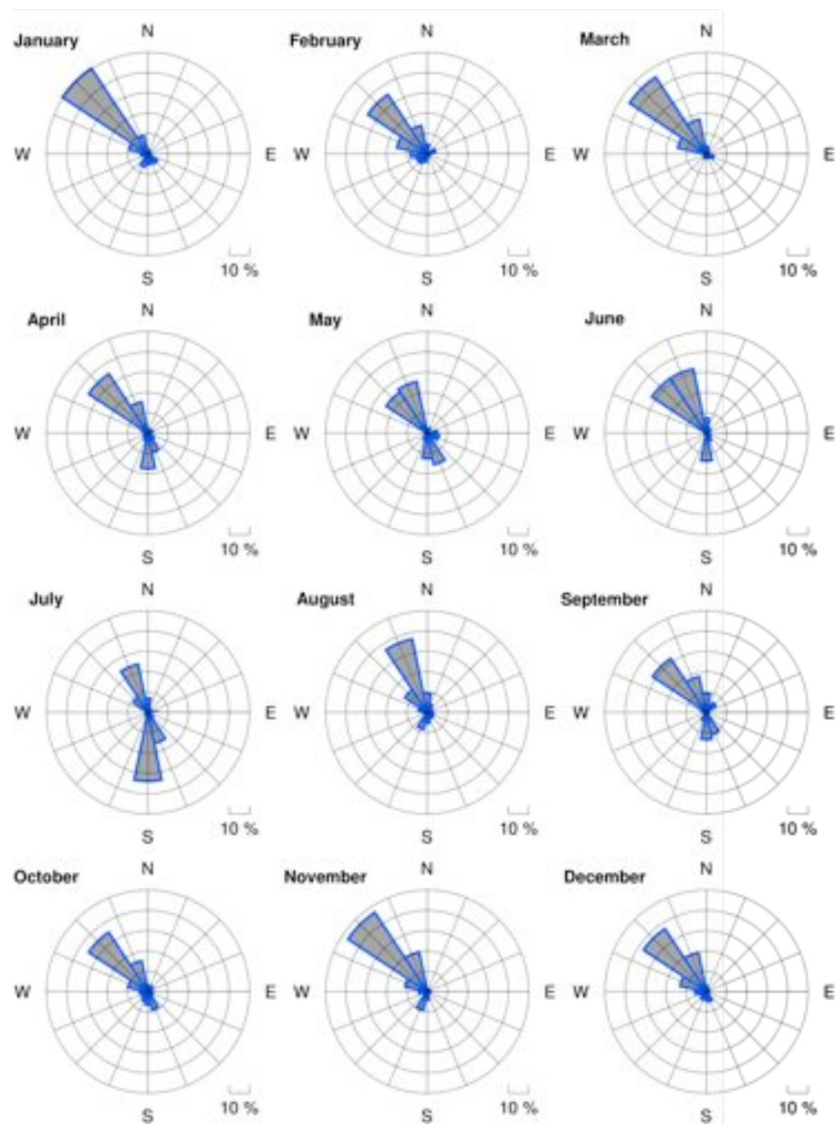
Figura III-58: Simulado en SLSI (San Ignacio de Velasco, Bolivia)
