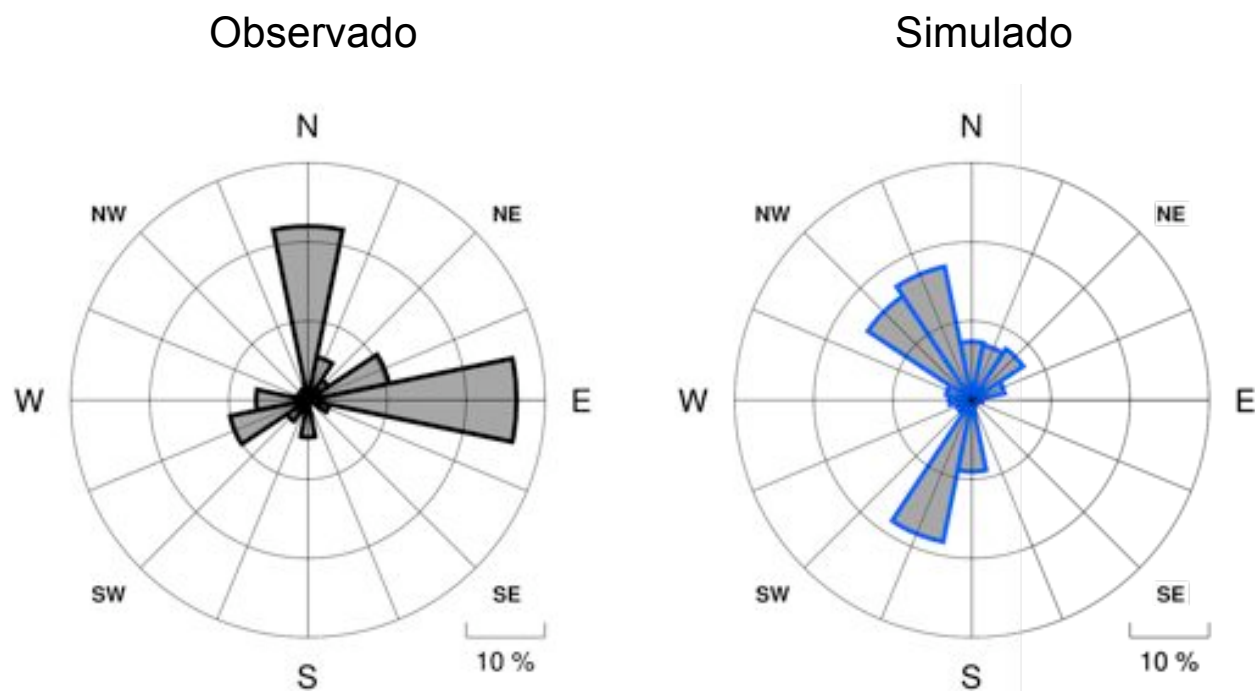
Figura III-13: Comparación Anual de Rosas de Viento: SLPS
