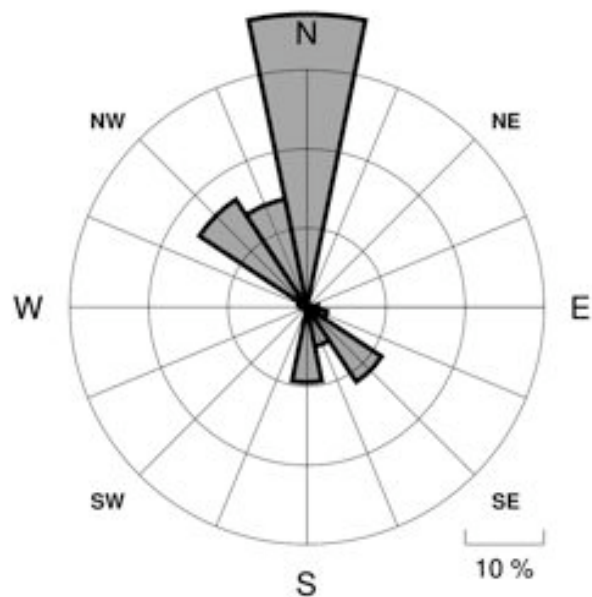
Figura III-9: Comparación Anual de Rosas de Viento: SLJO
