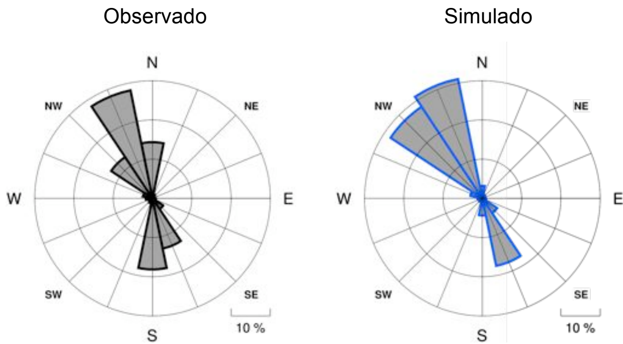
Figura III-21: Comparación Anual de Rosas de Viento: SLVR
