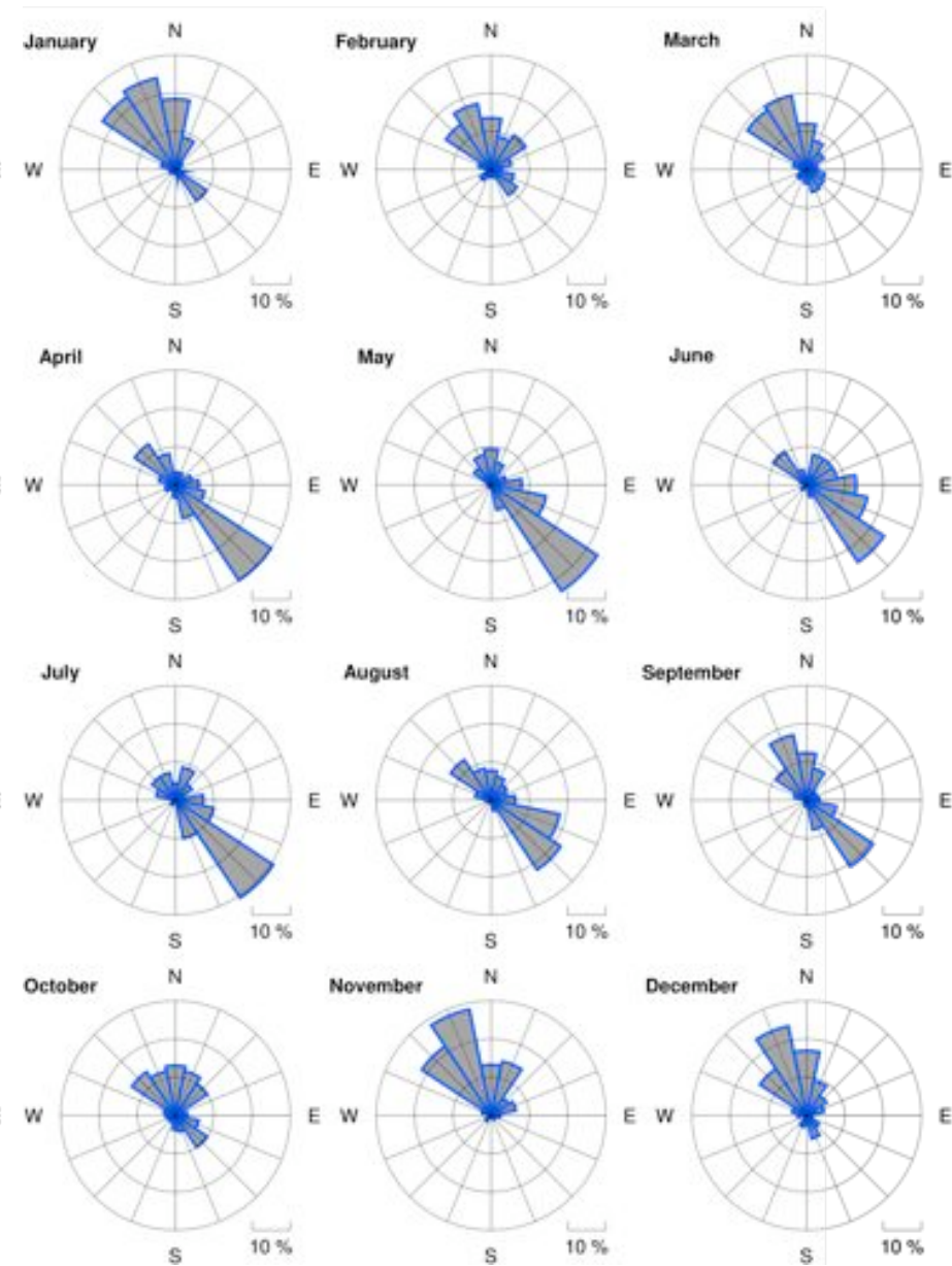
Figura III-32: Simulado en SLCO (Cobija, Bolivia)
