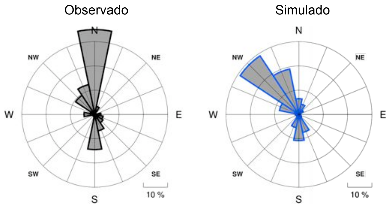
Figura III-8: Comparación Anual de Rosas de Viento: SLJE
