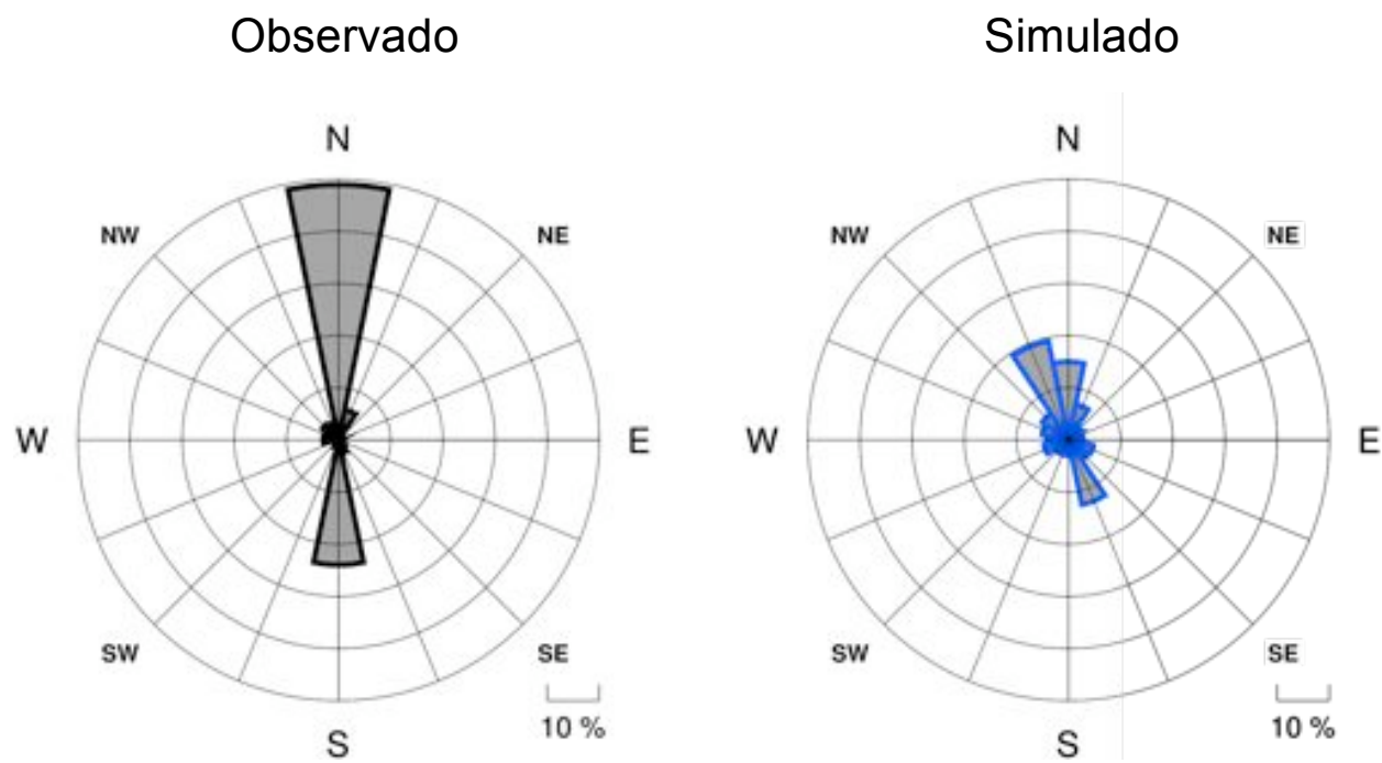
Figura III-15: Comparación Anual de Rosas de Viento: SLRI
