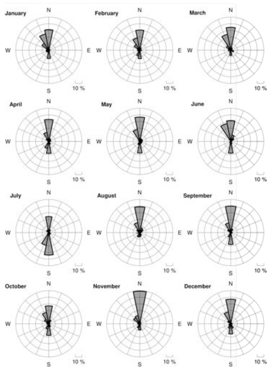
Figura III-57: Observado en SLSI (San Ignacio de Velasco, Bolivia)
