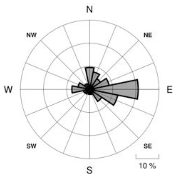
Figura III-10: Comparación Anual de Rosas de Viento: SLLP
