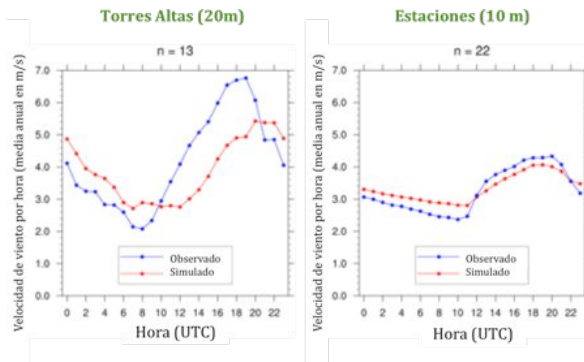
Figura 6: Ciclo diurno de la media de velocidad del viento por hora para datos simulados y observados de: velocidad del viento a 20 m en 13 torres altas (promedio de todas - izquierda) y velocidad del viento a 10 m en 22 estaciones meteorológicas (promedio de todos - derecha). La unidad de medida es metro por segundo (m/s).
