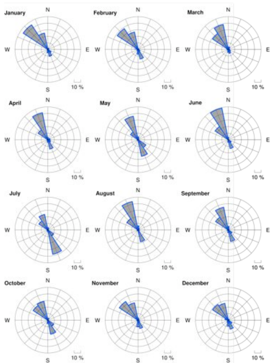
Figura III-36: Simulado en SLET (Santa Cruz / El Trompillo, Bolivia)
