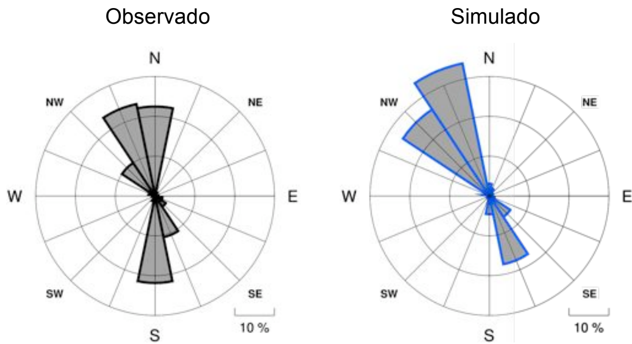
Figura III-7: Comparación Anual de Rosas de Viento: SLET
