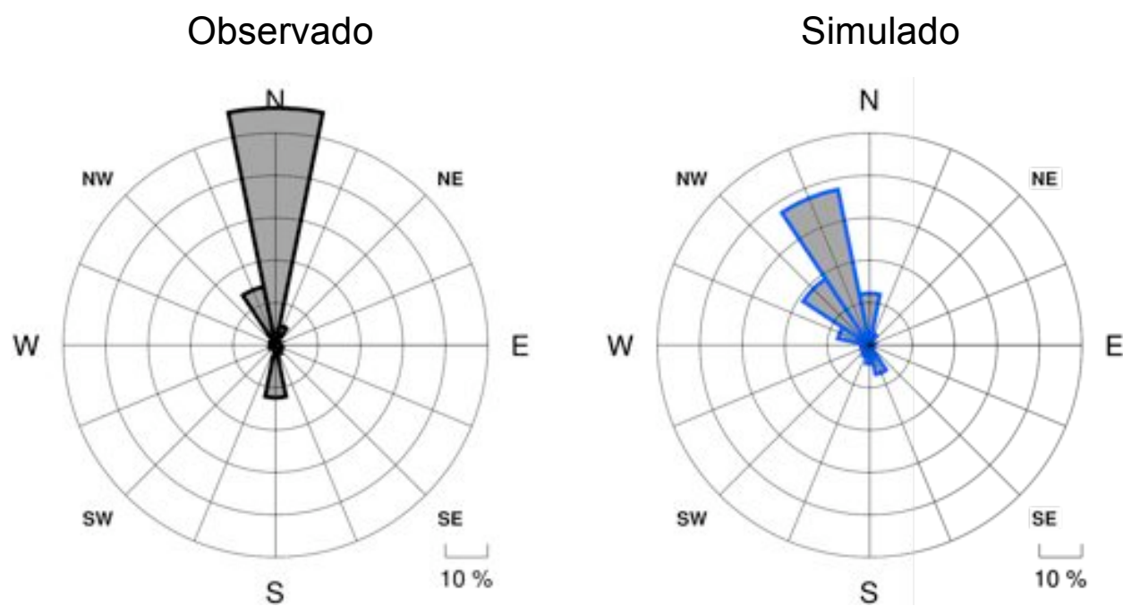
Figura III-14: Comparación Anual de Rosas de Viento: SLRB
