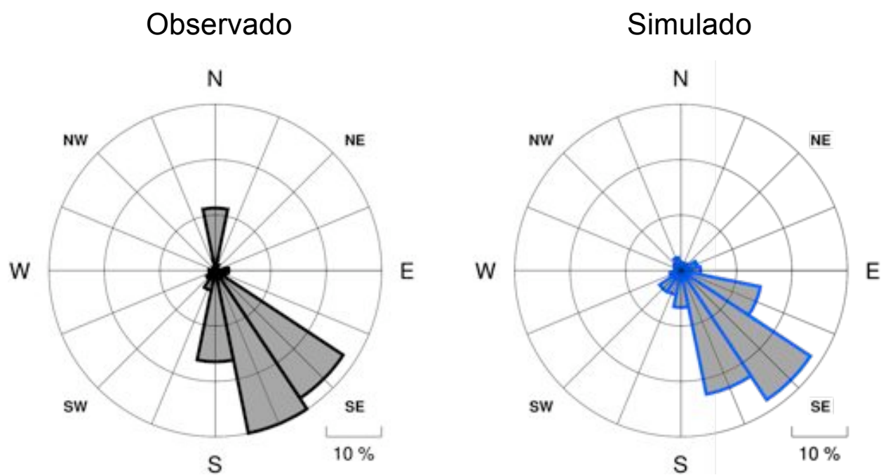
Figura III-20: Comparación Anual de Rosas de Viento: SLTJ
