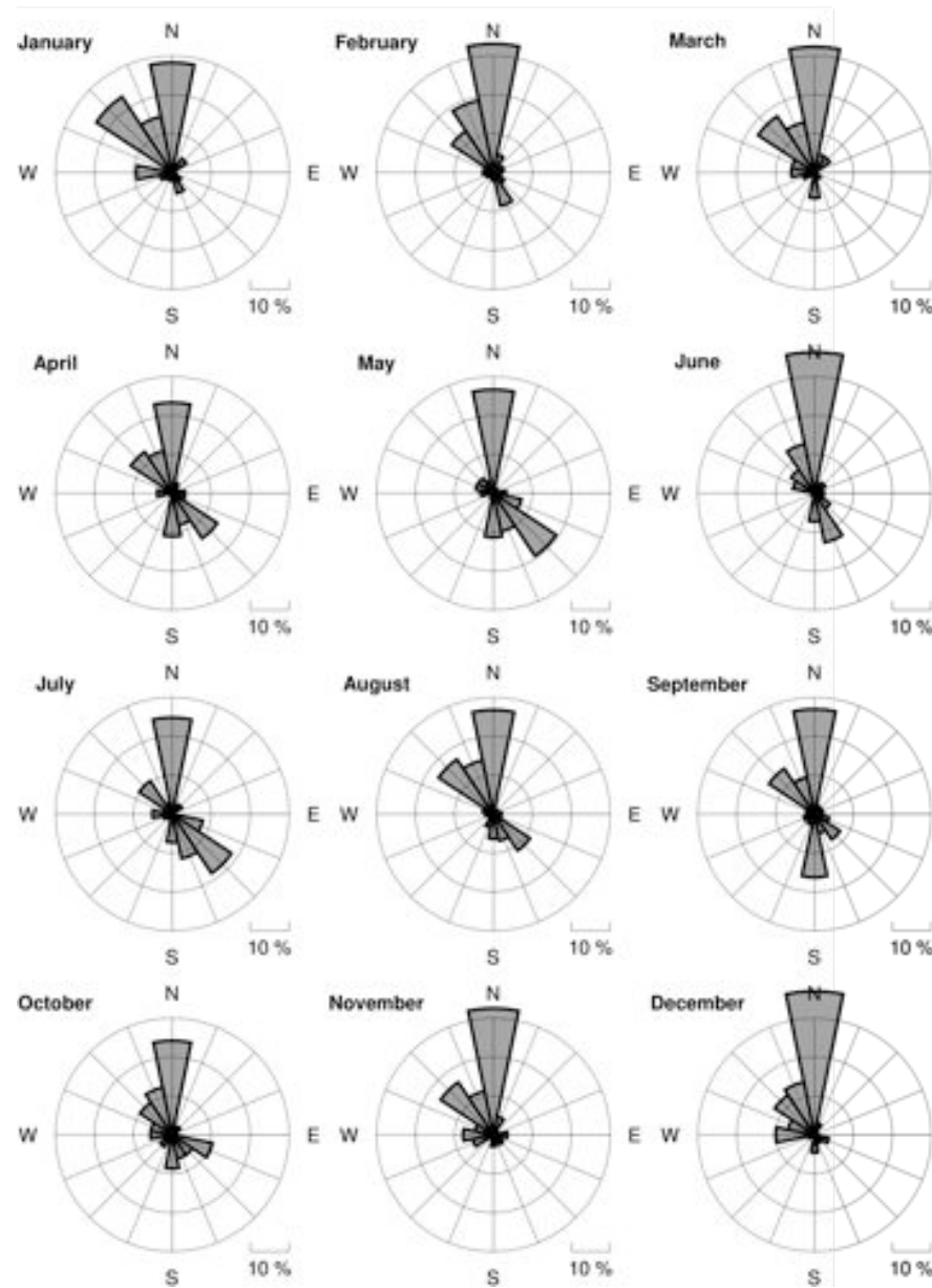
Figura III-31: Observado en SLCO (Cobija, Bolivia)
