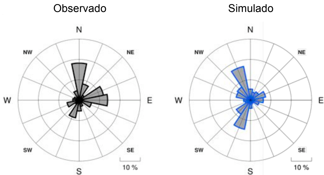
Figura III-1: Comparación Anual de Rosas de Viento: SBCR
