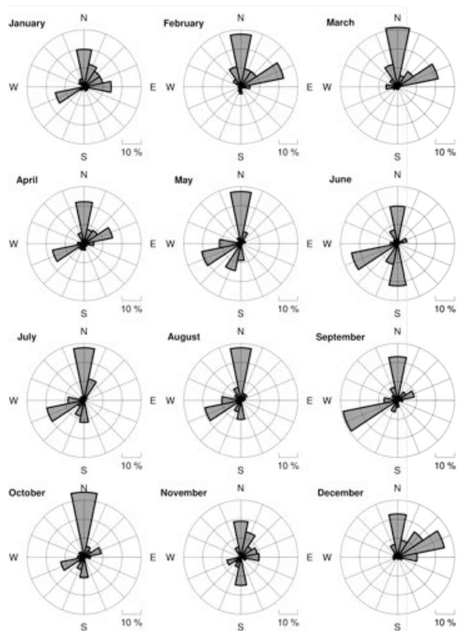
Figura III-45: Observado en SLPO (Potosí, Bolivia)
