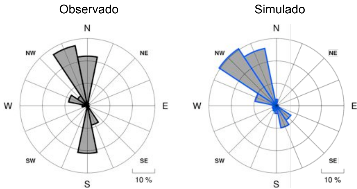
Figura III-6: Comparación Anual de Rosas de Viento: SLCP
