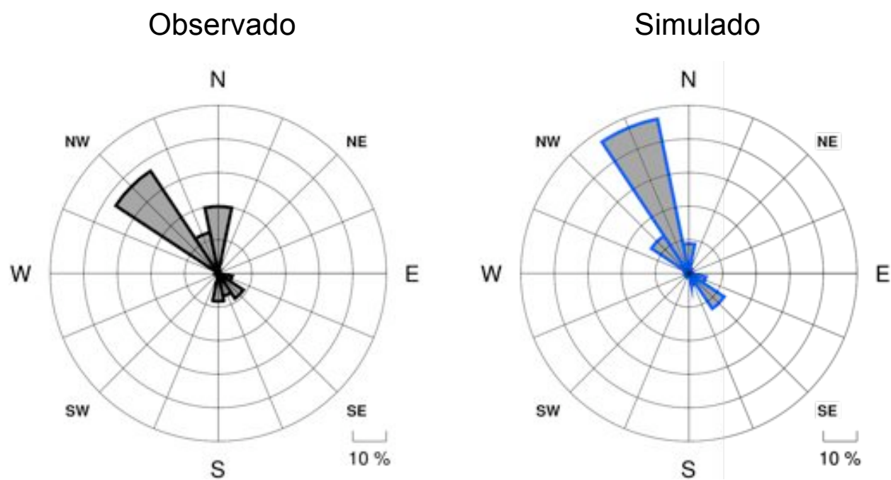
Figura III-16: Comparación Anual de Rosas de Viento: SLRY
