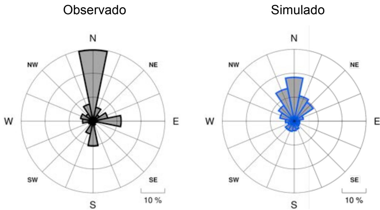
Figura III-11: Comparación Anual de Rosas de Viento: SLOR
