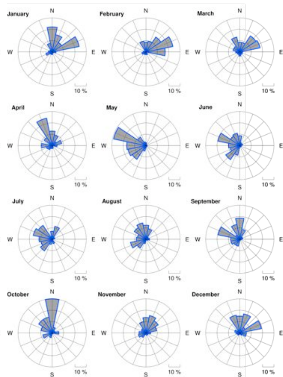
Figura III-46: Simulado en SLPO (Potosí, Bolivia)
