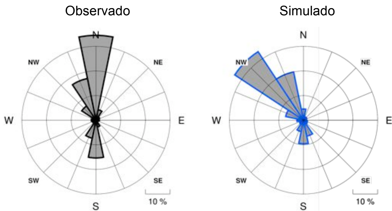
Figura III-18: Comparación Anual de Rosas de Viento: SLSI
