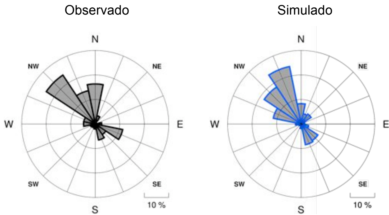
Figura III-17: Comparación Anual de Rosas de Viento: SLSA
